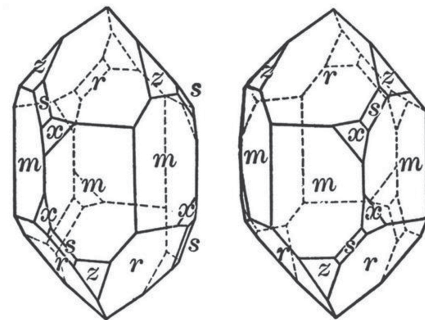
Рисунок – Левосторонняя хиральность в кристаллах кварца Figure – Left-handed chirality in quartz crystals
